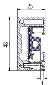
GS 25 STYRFÄSTE MED VÄGGFÄSTE
