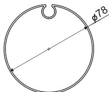
RULLRÖR
