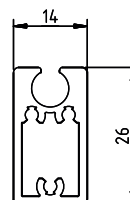
BOTTENSTÄNG
